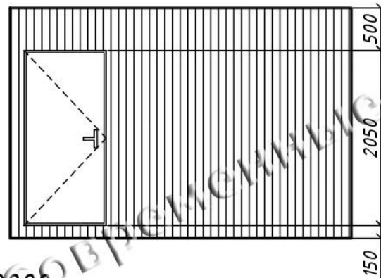
ТЫЛЬНАЯ
