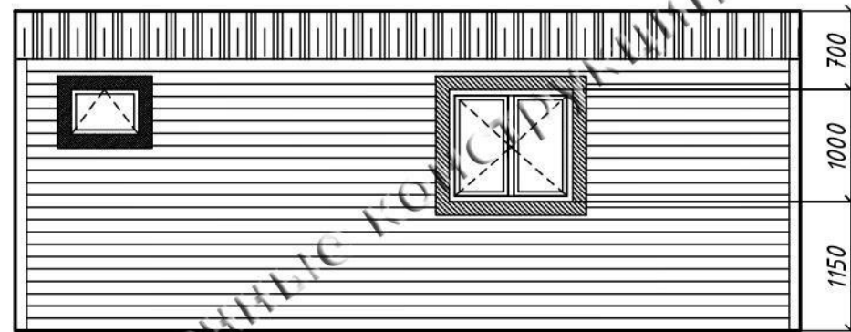
ЛЕВАЯ ТОРЦЕВАЯ
