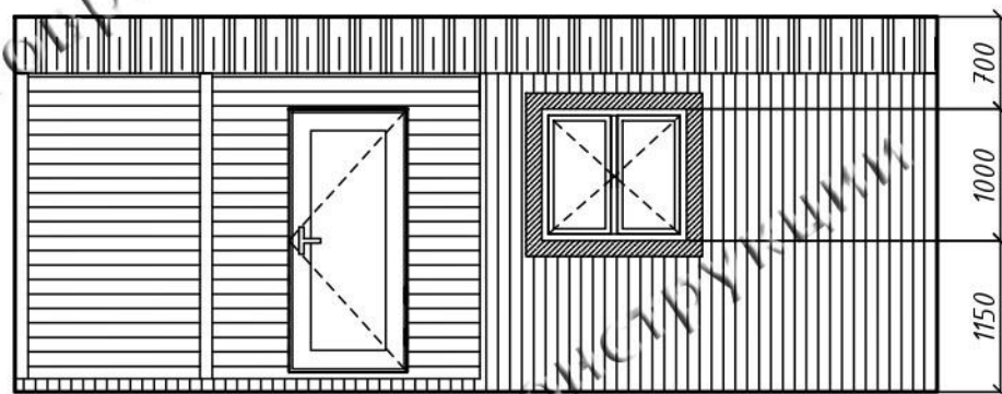
ТЫЛЬНАЯ
